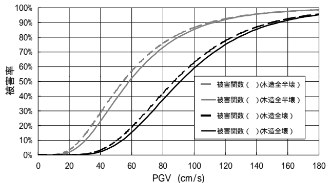
図 19 建物被害関数( )と( )の比較（木造）
