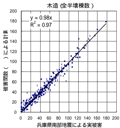
図 18 建物被害関数( )と( )による町丁目ごとの推定被害棟数と実被害との比較
